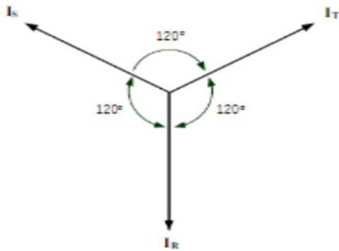
Gambar 3.1 Diagram Vektor Arus Keadaan Seimbang
